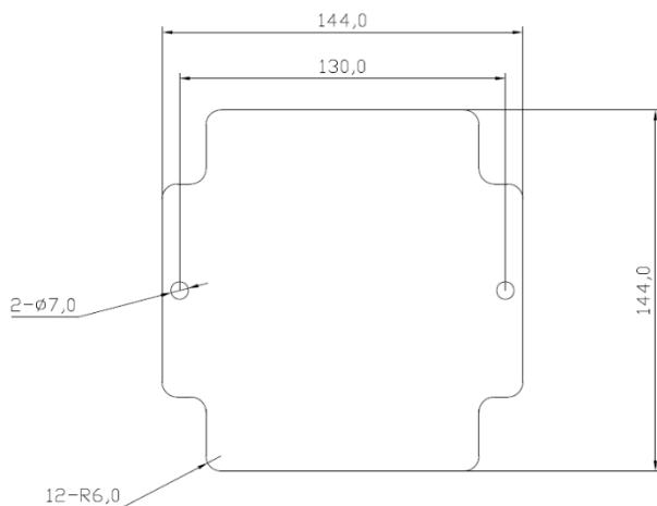
PM-CRADYBOX-AL-160X160X90 - 0186105
