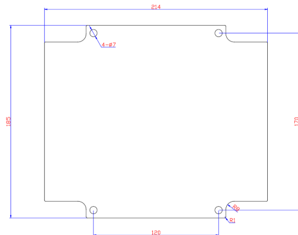
PM-CRADYBOX-AL-230X200X110 - 0186107
