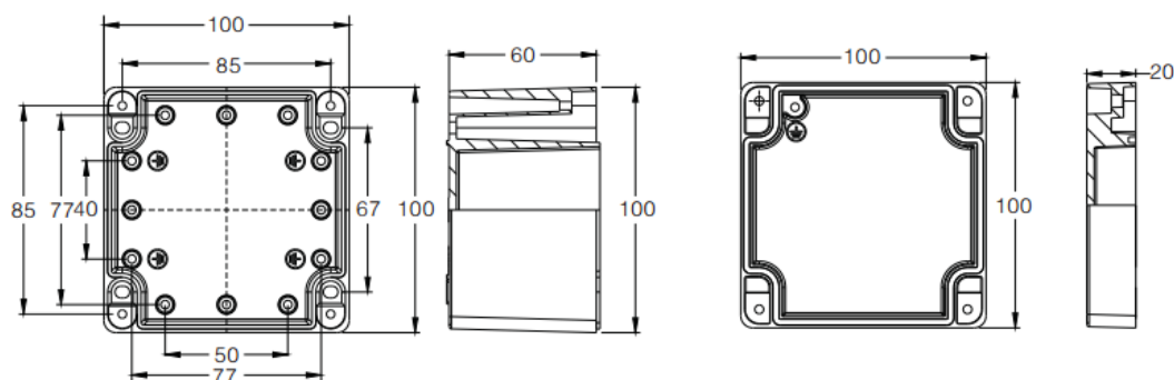
CRADYBOX-AL-125X125X80 - 0186003
