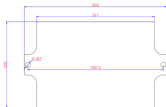
PM-CRADYBOX-AL-220X140X90 - 0186106
